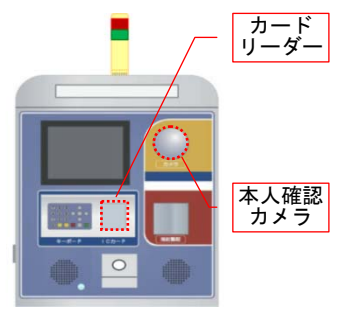
図1 リーダー筐体
